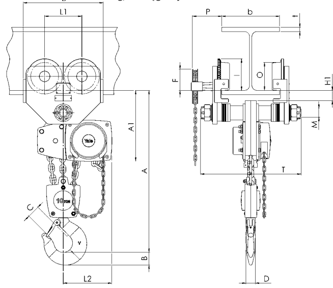
Model Yalelift ITP/ITG 5.000 kg, dwuciągowy
