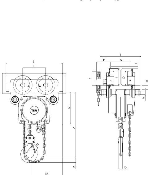
Model Yalelift ITP, 500 - 3.000 kg, z jednym ciągnem
