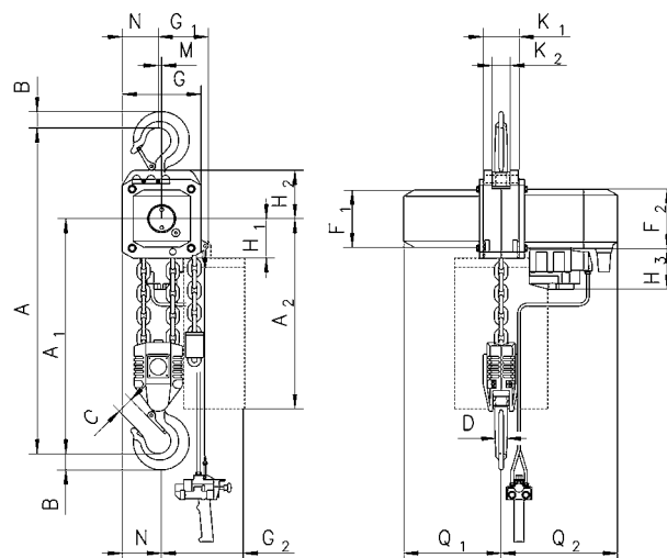
Model CPA z hakiem zaczepowym, 4.000 - 6.000 kg, dwuciągnowy
